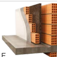
DOBLE PARED CON AISLAMIENTO LLENANDO PARCIALMENTE LA CÁMARA DE AIRE
