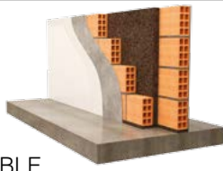
DOBLE PARED CON AISLAMIENTO LLENANDO TOTALMENTE LA CÁMARA DE AIRE
