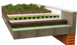
CUBIERTA PLANA AJARDINADA
